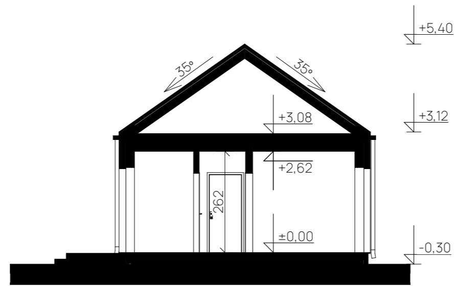
PRZEKRÓJ A-A
