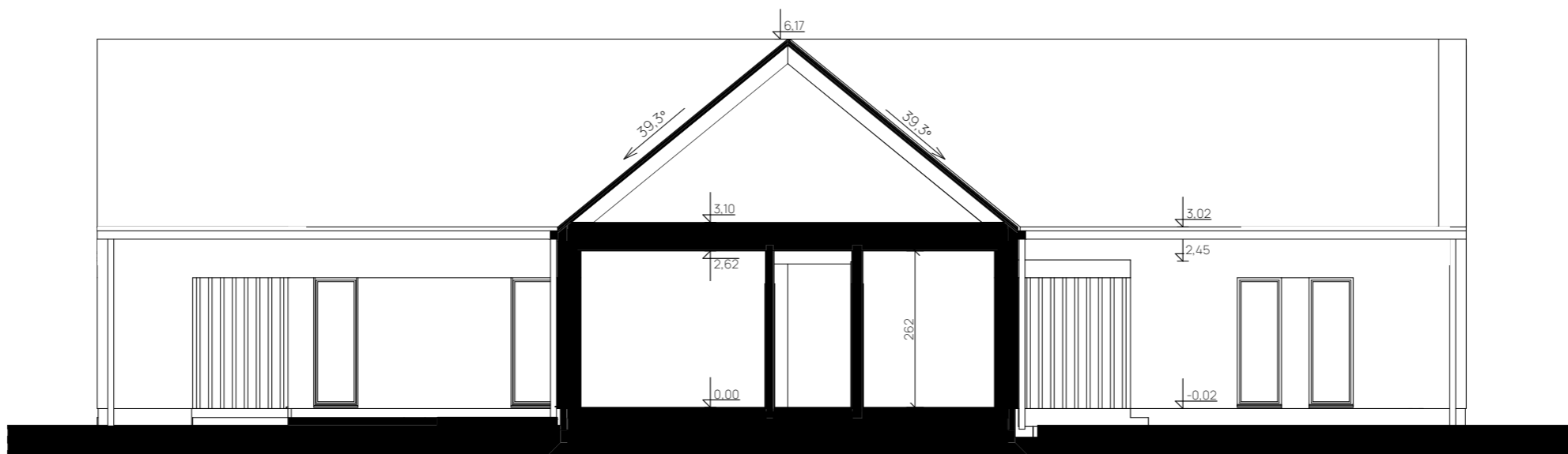
PRZEKRÓJ A-A
